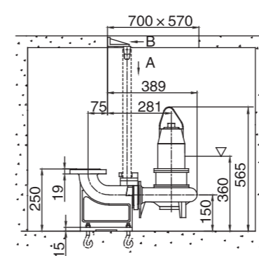
Z — монтаж с использованием крепеж-захвата
