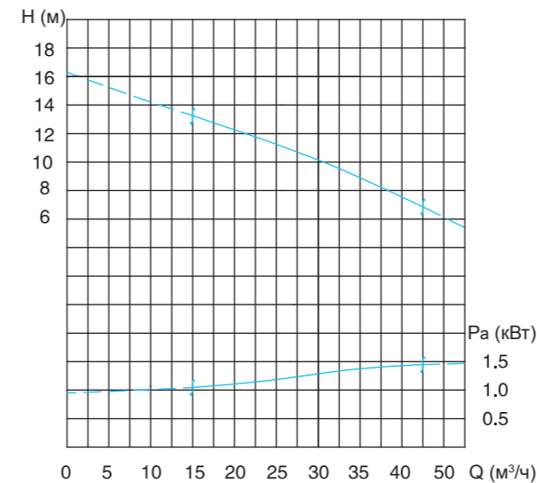
Кривая производительности
