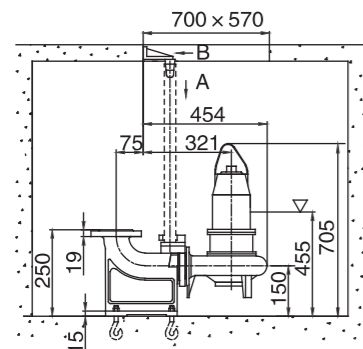
Z — монтаж с использованием крепеж-захвата
